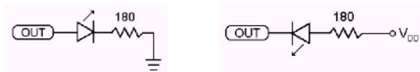
Dos posibles formas de conectar un led
